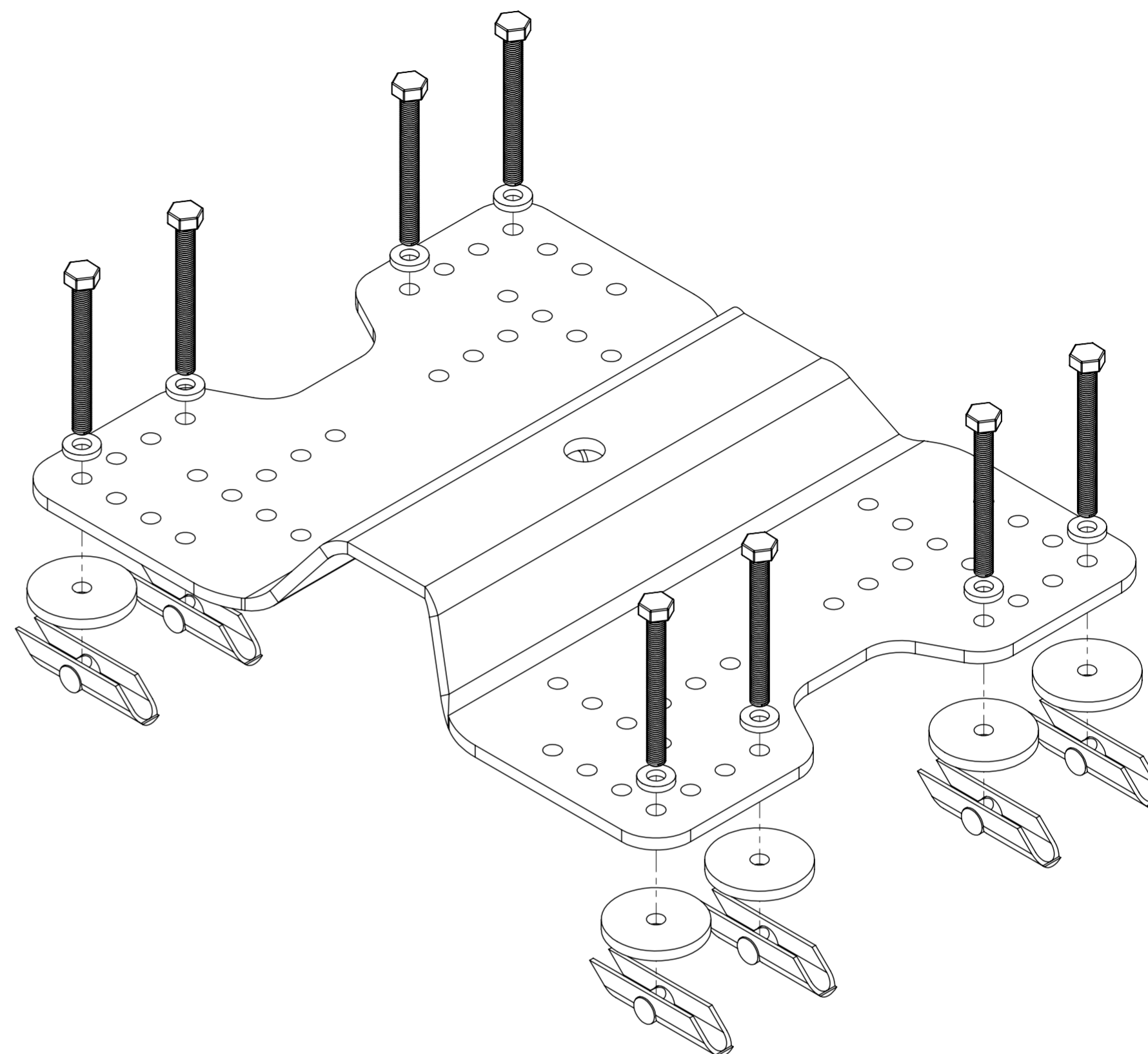
Vue éclatée
